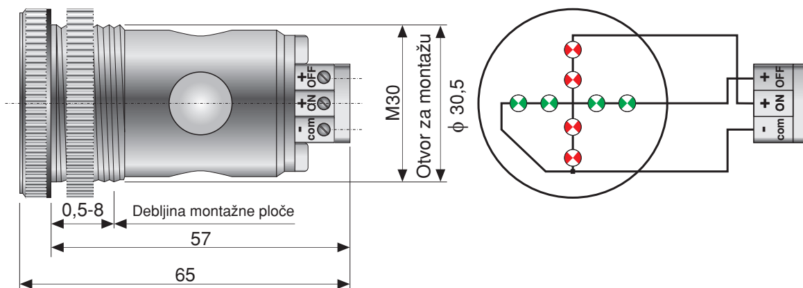
Merna skica pokazivača položaja MPP-1
